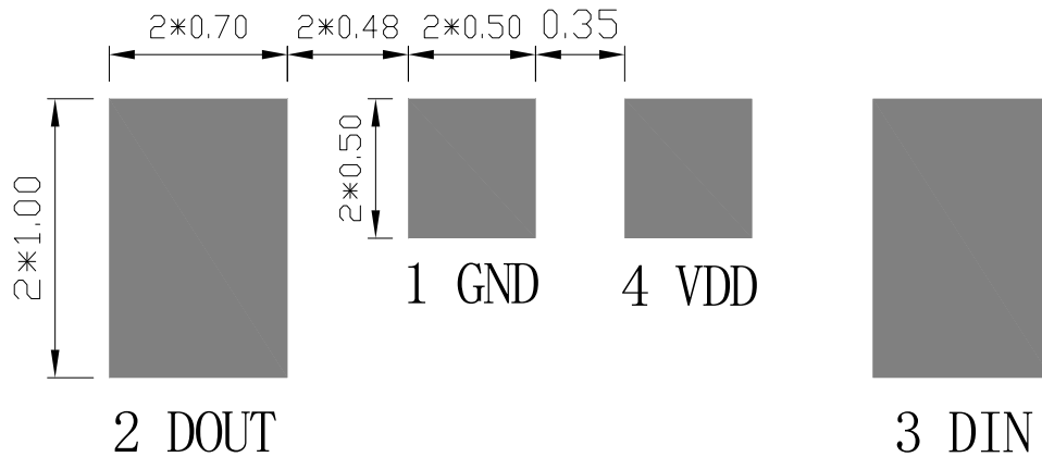
侧面贴装建议焊盘尺寸
