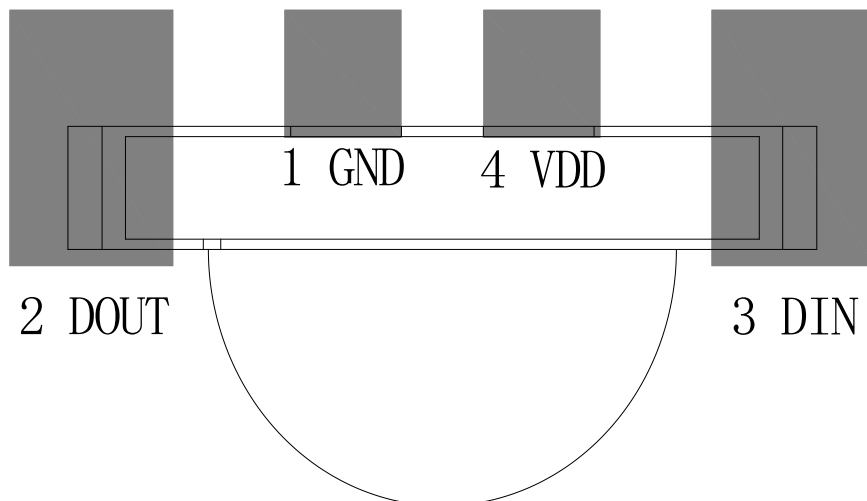
侧面贴装示意图
